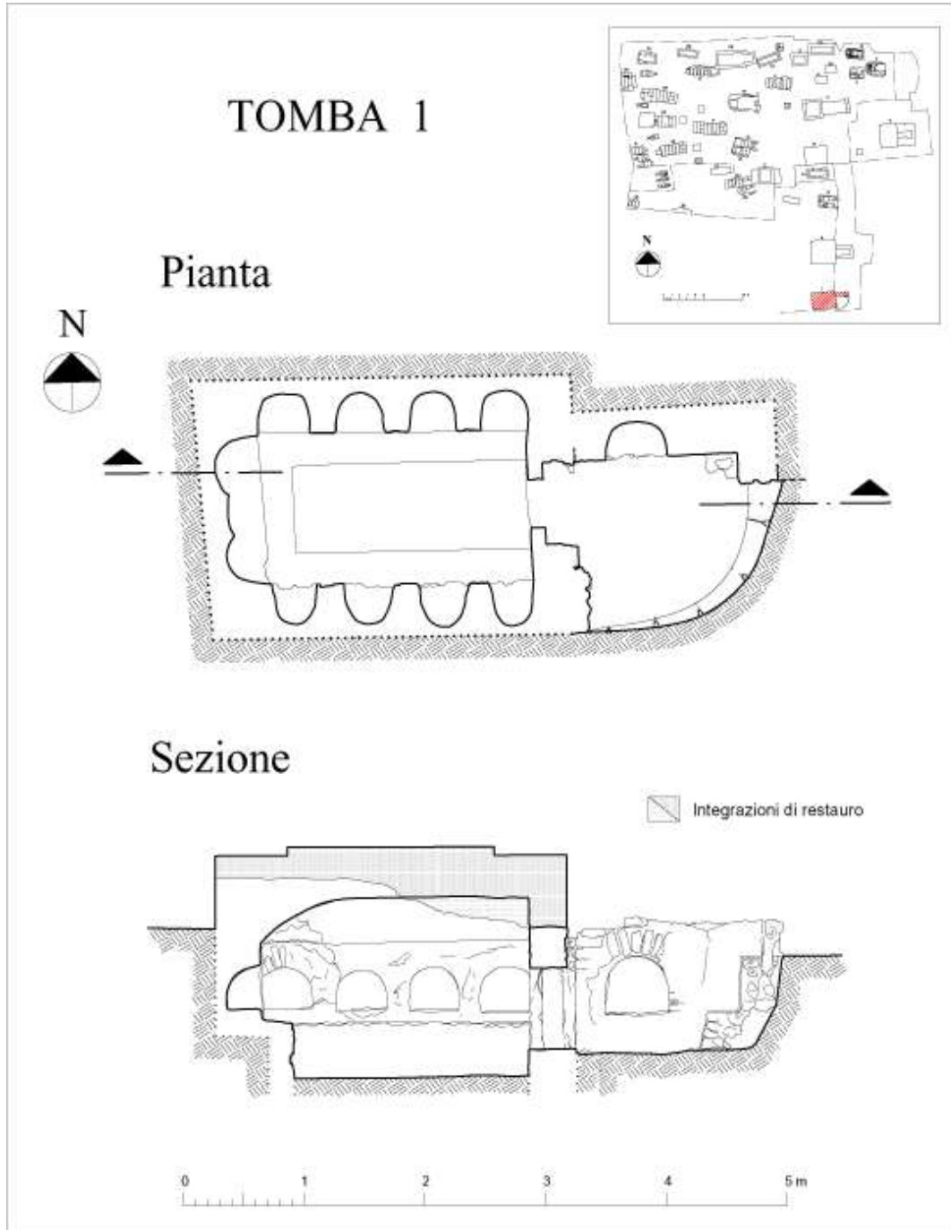
خريطة ومسقط للمدفن رقم (1)
