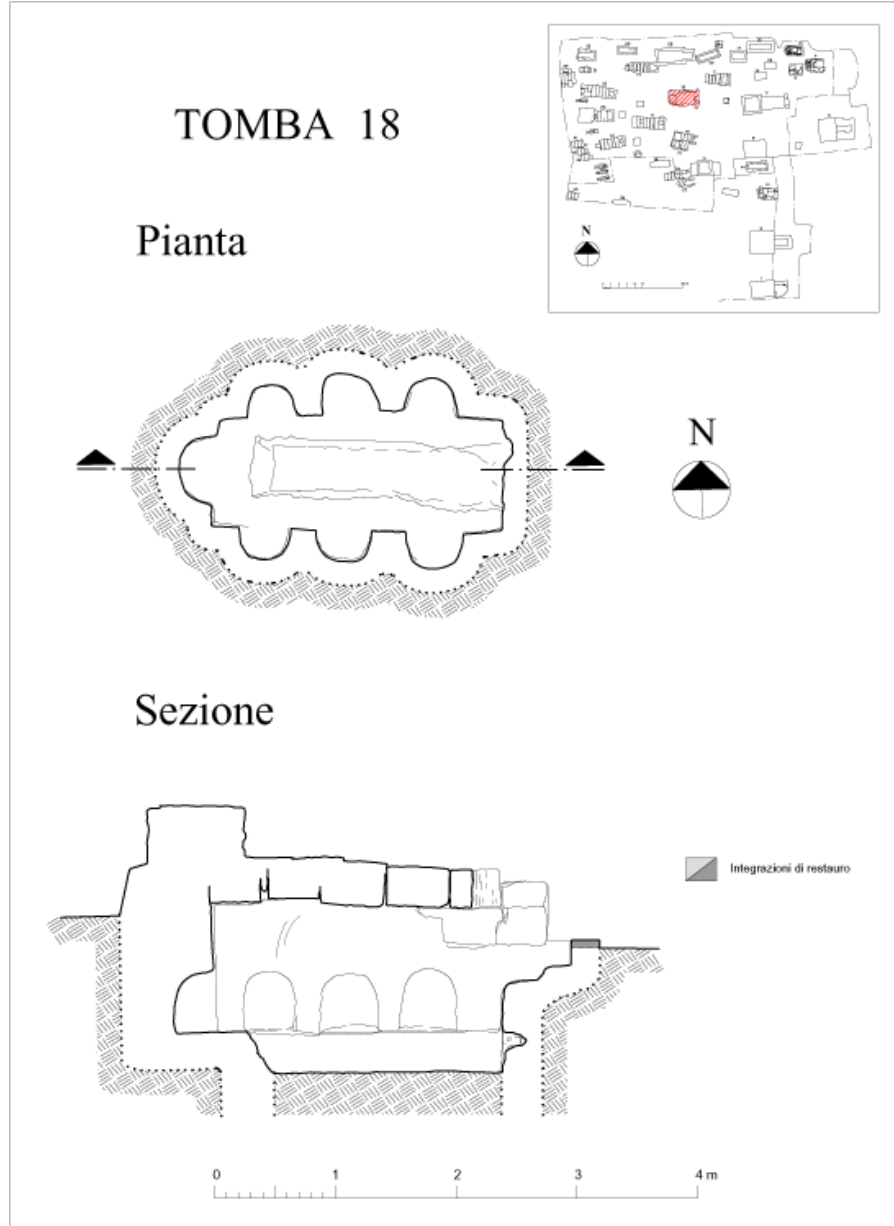
خريطة ومسقط للمدفن رقم (18)
