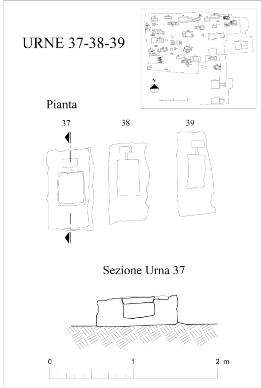
خريطة ومسقط للمدافن (37 ، 38 ، 39)
